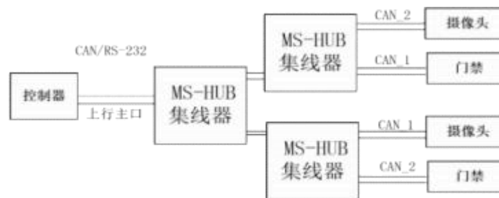
级联扩展接法
