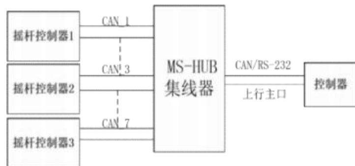
反向接法
